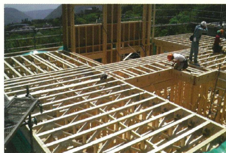
●2階床にトラス使用の「住宅」
